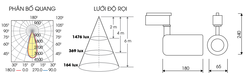
TRL06 20W
