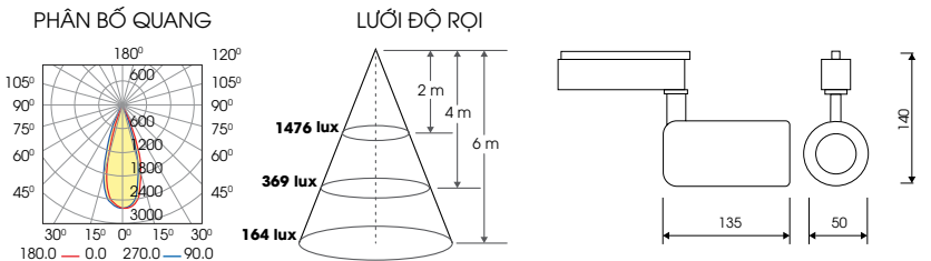
TRL05 20W
