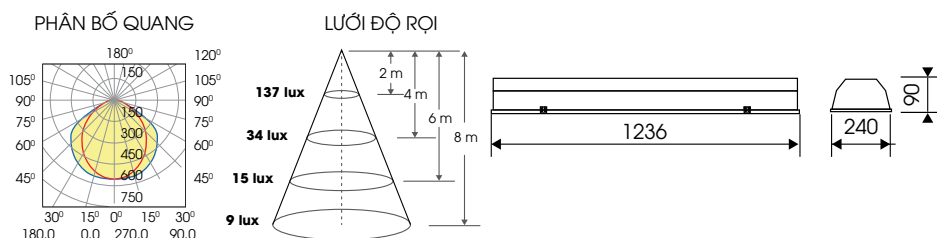
T8 CSLH/20Wx2
