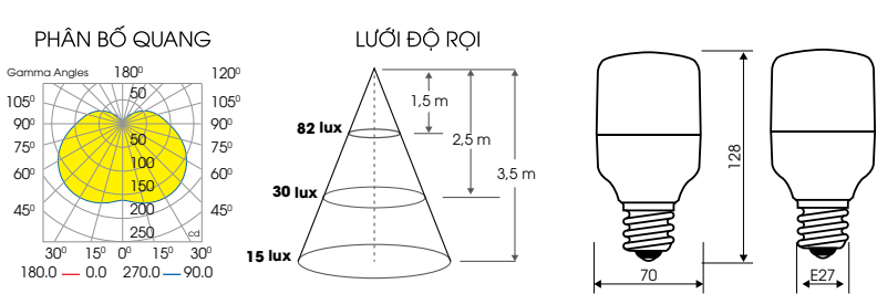
TR70N1/14W.H
