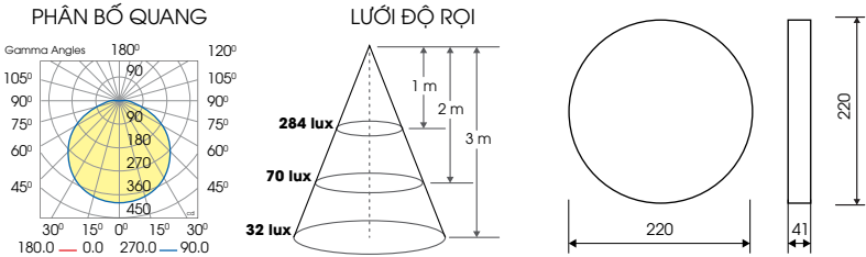
LN12N 220x220/18W
