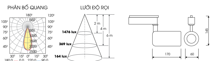
TRL05 30W
