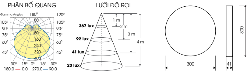
LN12N 300/24W
