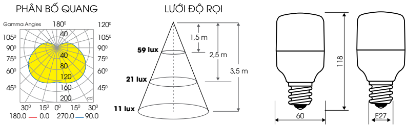
TR60N2/10W.H
