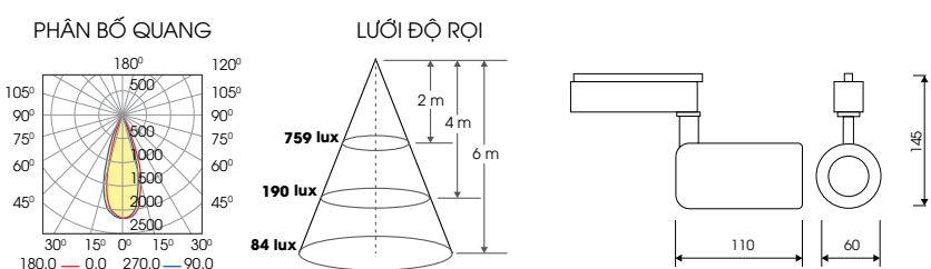
TRL05 20W
